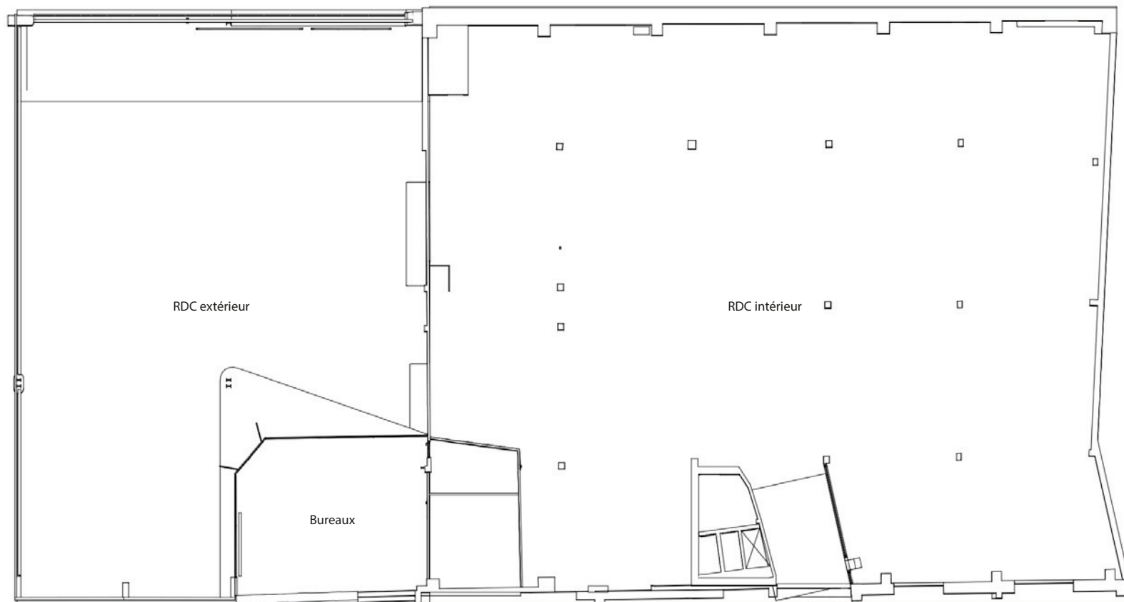
PLAN RDC
